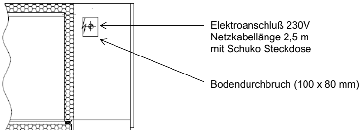
Bild 4: Draufsicht Kühltsch (Zentralkühlung)
