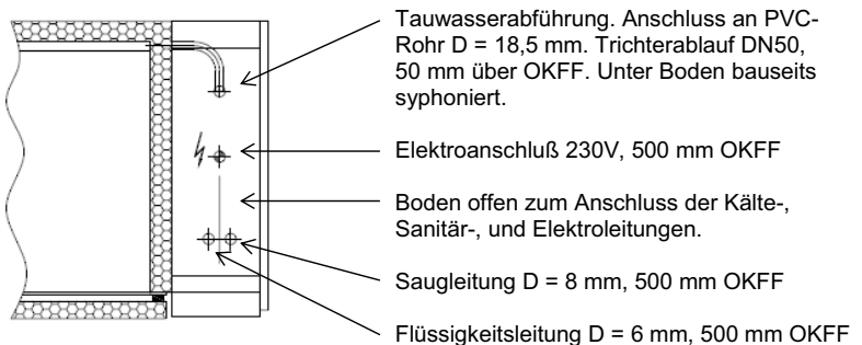
Bild 4: Draufsicht Kühltsch (Zentralkühlung)
